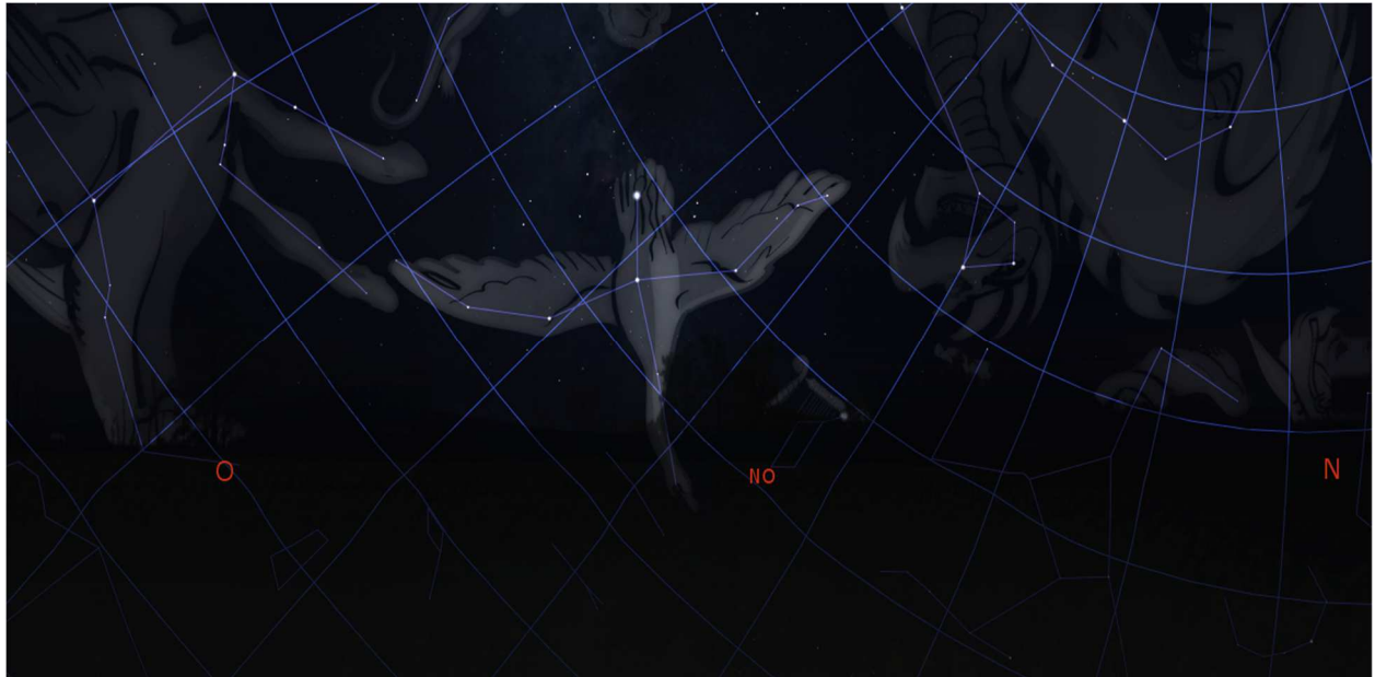
Figura 4. Nello stesso momento in cui Fetonte cade nell'Eridano, il Cigno tuffa la sua testa sotto l'orizzonte tramontando a nord-ovest.
